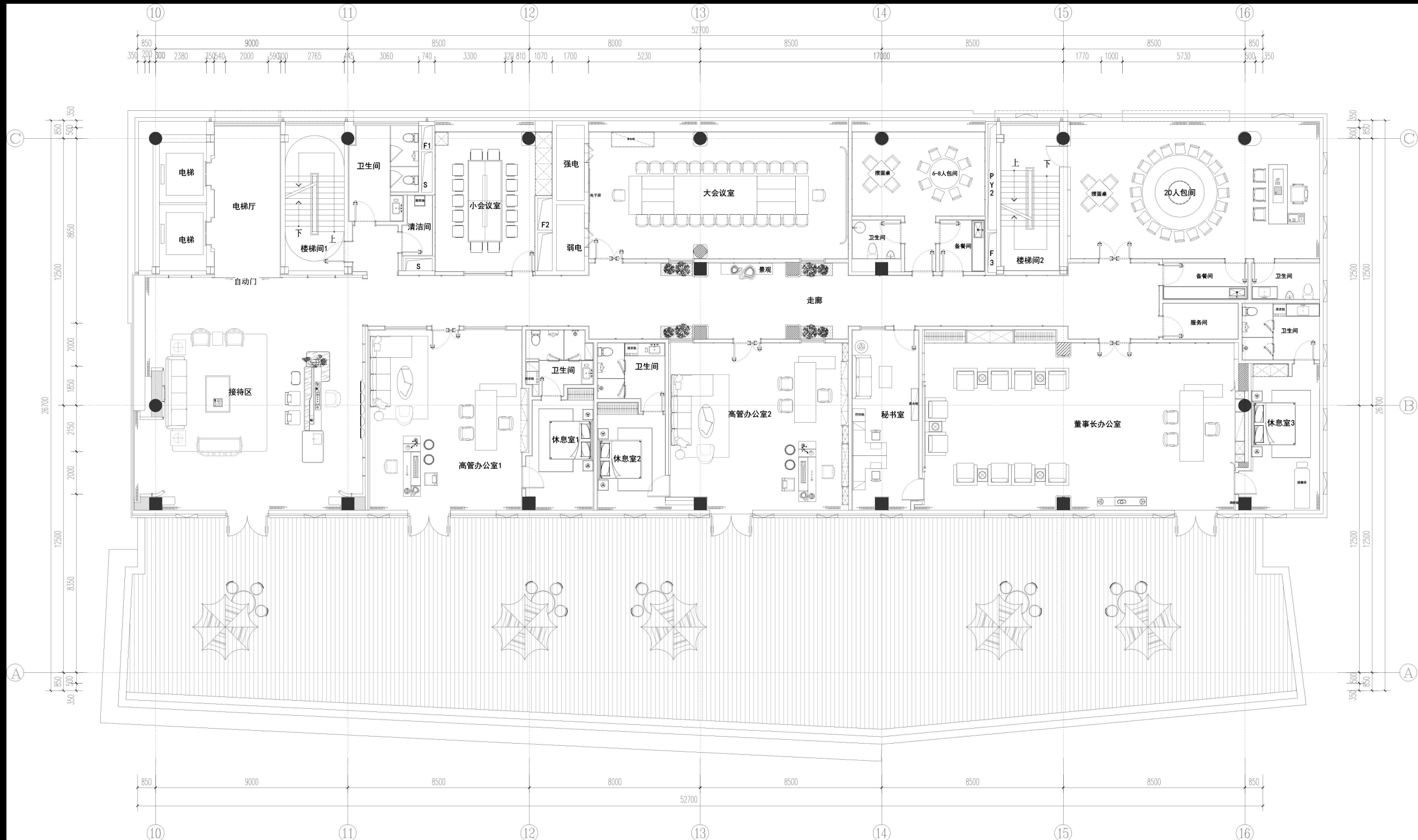
- 5F平面布置图 - 5F FLOOR PLAN
