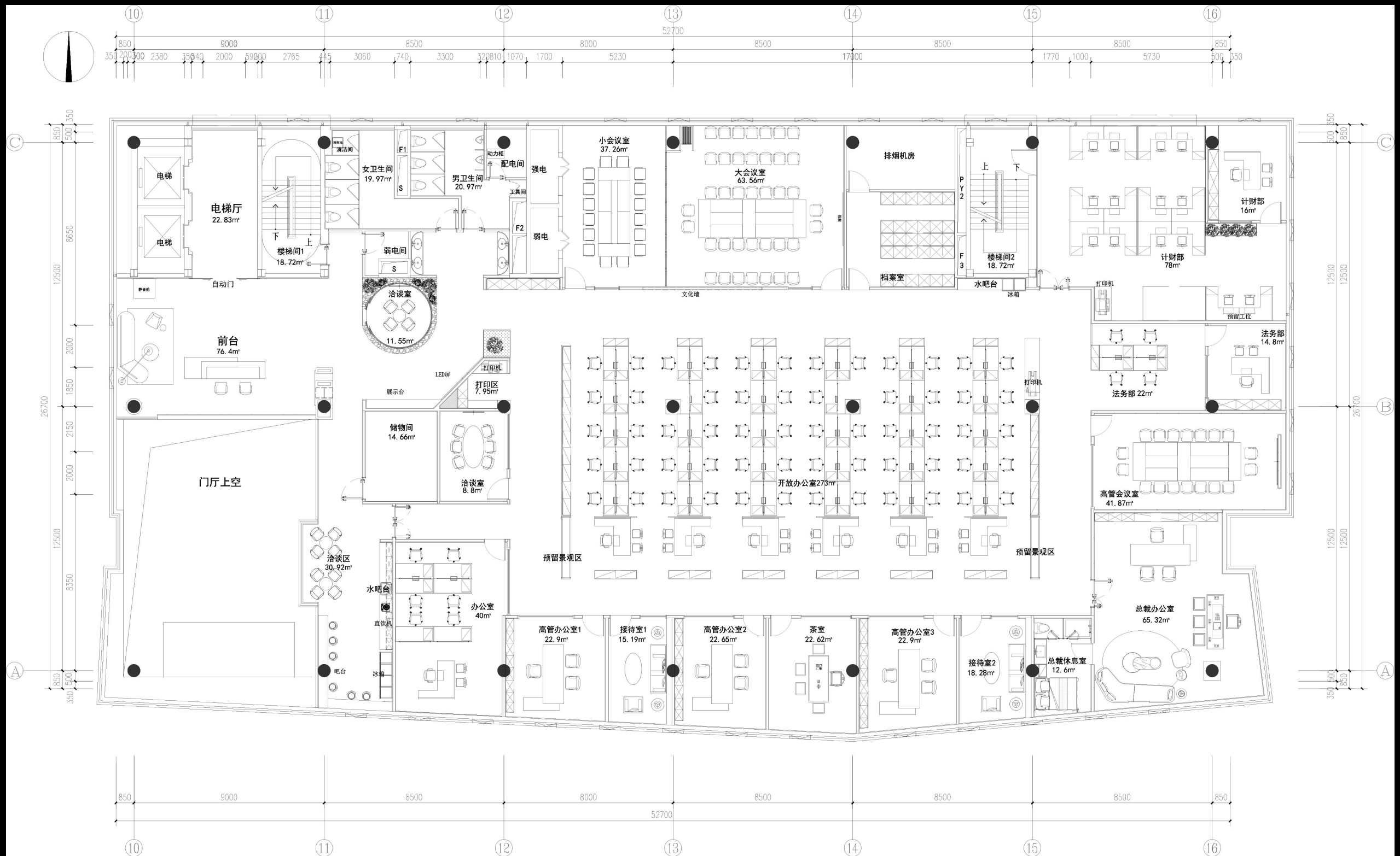
- 4F平面布置图 - 3F FLOOR PLAN
